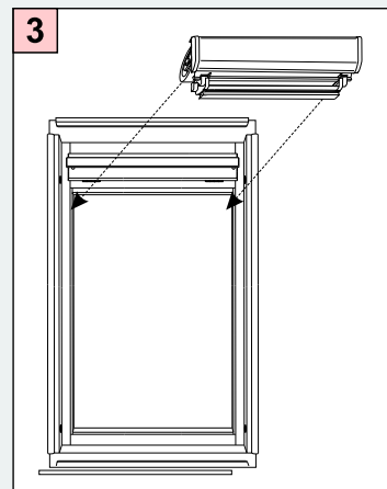
Montaż kasety
