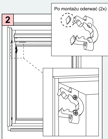
Umocowanie uchwytu
