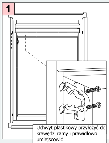
Umiejscowienie uchwytu
